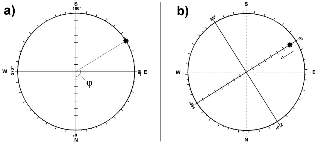
Abb. 6.5 Das Prinzip der indirekten Kometennachführung unter Verwendung eines Fadenkreuzokulars mit Teilstreichen und Winkelskala (ohne Zenitprisma) am Beispiel eines Bewegungswinkels \varphi von 122^\circ : a) Einstellung des Bewegungswinkels auf der Winkelskala, b) Ausrichten der Strichskala und Bewegen des Leitsterns in definierten Schritten entgegengesetzt zur Bewegungsrichtung des Kometen
