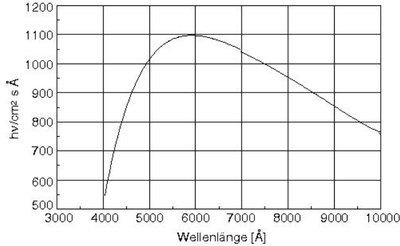
Abb. 7.13 Zahl der Quanten in \text{cm}^{-2} \text{s}^{-1} \text{\AA}^{-1} für einen G2-Stern der 0. Größe außerhalb der Atmosphäre
