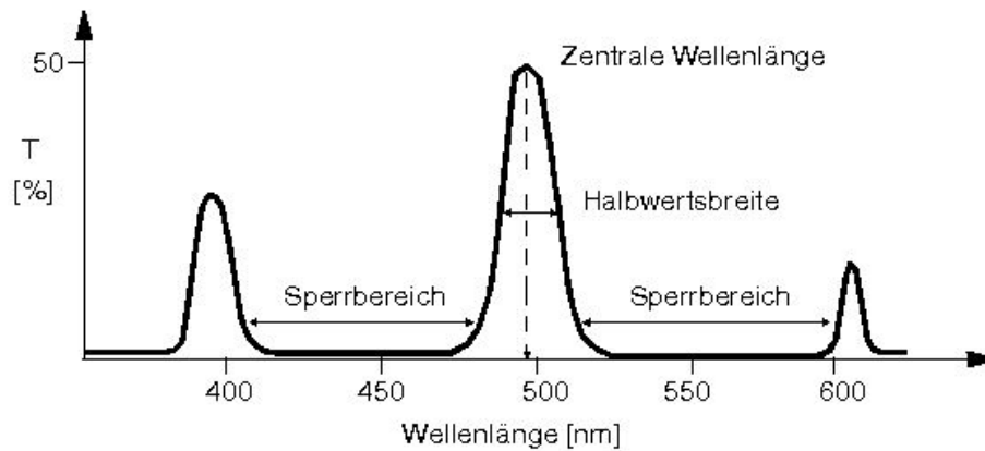
Abb. 7.20 Schematische Darstellung von Transmissionskurven verschiedener Ordnungen eines Interferenzfilters. T: Transmission
