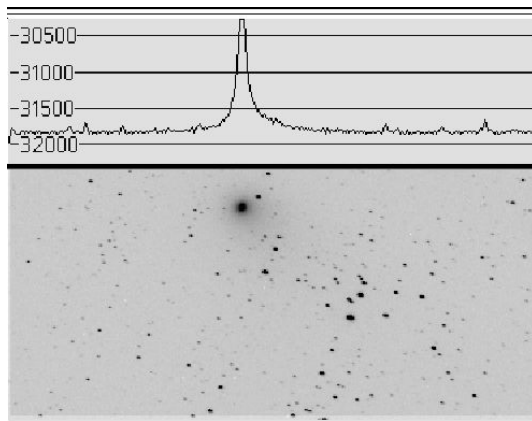
Abb. 7.27 Festlegung der Diaphragmagröße mit Hilfe eines xz-Querschnitt-Plots ( Imagine-32 )
