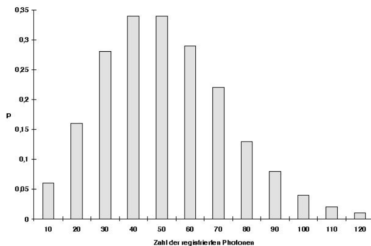
Abb. 7.12 Beispiel einer Poisson-Verteilung mit der Varianz \sigma^2 = 50 für die Zahl registrierter Photonen
