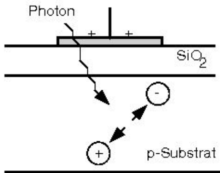
Abb. 7.3 Schematischer Aufbau eines MOS-Kondensators
