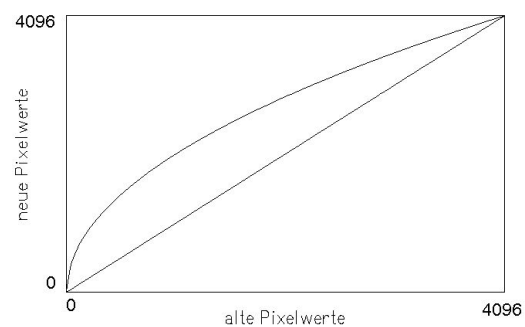
Abb. 7.33 Skalieren mit Potenzgesetzen; Exponent p = 0.5
