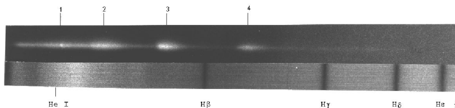
Abb. 9.3 Photographisches Spektrum des Kometen C/1996 B2 (Hyakutake). Die Aufnahme wurde mit einem Objektivprisma gewonnen: das Prisma sitzt vor dem Teleskop, das somit als Abbildungsoptik dient. Der Kollimator entfällt, da das Sternlicht bereits parallel ist. Von links nach rechts erkennt man (in Klammern steht der nach Wellenlänge und Intensität aus Brown et al. (1996) wahrscheinlichste Wert für \lambda in nm): 1.) H_2O^+ (584.1) o. C_2 (583.9), 2.) C_2 (549.7), 3.) C_2 (510.1), 4.) C_2 (465.6). Darunter befindet sich ein Eichspektrum von ff Lyr, das für die Wellenlängenkalibrierung (Polynom 3.Grades) benutzt wurde. Instrument: Zeiss-Meniscas 180 mm f/10, Objektivprisma BK2 mit 45^\circ brechendem Winkel und 110 mm Kantenlänge. Am 15.04.1996 auf Kodak T-Max 3200 10 min belichtet. Photo: B.Hanisch (Frankfurt/Oder).
