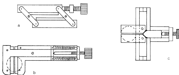
Abb. 9.5 Einige Varianten eines beweglichen Rasierklingspaltes. Nicht überall sind Federn eingezeichnet, welche die beweglichen Teile zusammenziehen. Varianten a) und b) öffnen unsymmetrisch, Variante c) öffnet symmetrisch. Zeichnung: K.-H. Uhlmann (Lampertheim).
