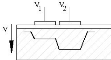
Abb. 7.6 Ladungskopplung zweier Potentialsenken
