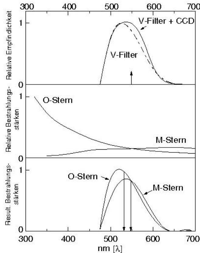
Abb. 7.19 Normierte Empfindlichkeitskurven. Oberes Diagramm: Resultierende spektrale Empfindlichkeitskurve aus V-Filter und CCD (TC-211). Mittleres Diagramm: Relative spektrale Energieverteilungen eines O- bzw. eines M-Sterns. Diagramm unten: normierte Netto-Bestrahlungsstärken. Im oberen Diagramm ist schematisch die effektive Wellenlänge (Pfeil nach oben) angegeben. Im unteren Diagramm sind die resultierenden quasi-isophoten Wellenlängen schematisch dargestellt
