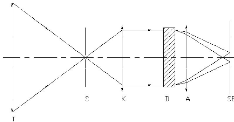
Abb. 9.1 Funktionsweise eines Spalt-Spektrographen. Teleskop T, Spaltblende S, Kollimator K, Dispersionselement D, Abbildungsoptik A, Strahlungsempfänger SE.
