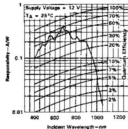
Abb. 7.11 Spektrale Empfindlichkeit des TC-211-Bausteins von Texas Instruments
