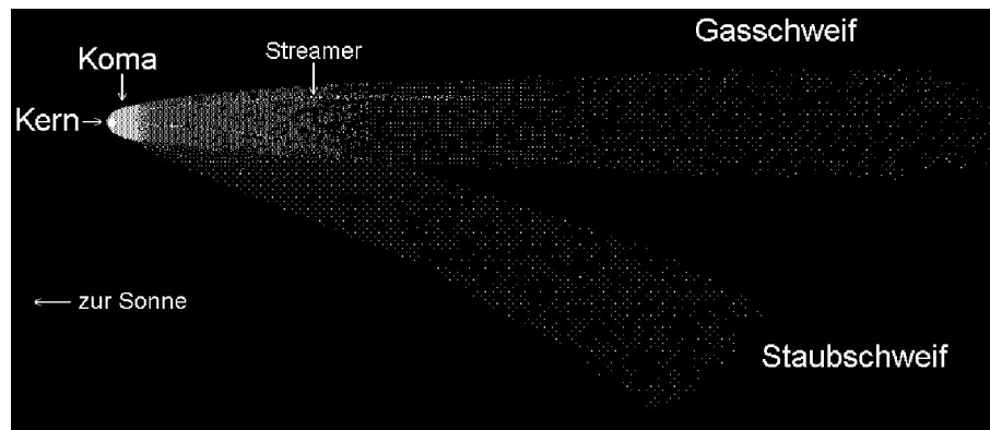
Abb. 1.1 Schematische Darstellung eines Kometen (A. Kammerer)
