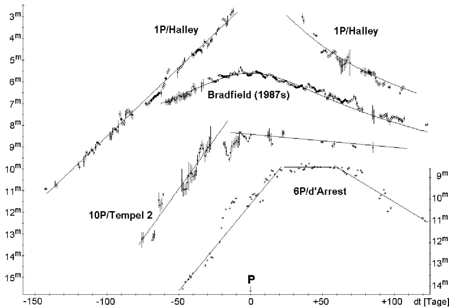
Abb. 5.5 Die heliozentrische Helligkeit von vier ausgewählten Kometen, aufgetragen über dt . Der Vergleich mit Abb. 5.4 zeigt, daß die Kometen 10P/Tempel 2 und 6P/d'Arrest eine Abhängigkeit von dt zeigen, der Komet Bradfield (1987s) hingegen von \log r . Beim Kometen 1P/Halley konnte die Entwicklung 1985/86 vor dem Perihel besser mit einer dt -, nach dem Perihel besser mit einer \log r -Abhängigkeit beschrieben werden
