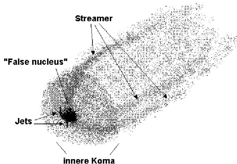
Abb. 3.9 Schematische Darstellung der inneren Kometenkoma
