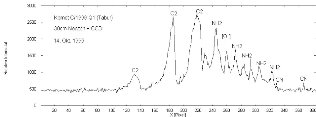
Abb. 9.10 Spektrum des Kometen C/1996 Q1 (Tabur) als Zeilenscan der Abb. 9.8. Aufgrund der kurzen Spektrumslänge ist die spektrale Auflösung relativ gering. Nur die intensivsten Emission-Banden wurden mit Hilfe des Linienkataloges von Brown et al. (1996) identifiziert.
