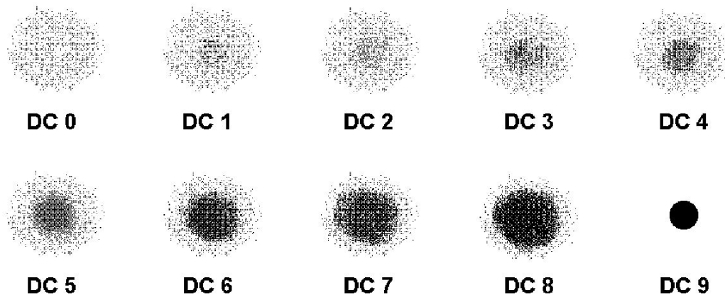
Abb. 3.8 Der Kondensationsgrad der Koma (kurz: DC).
