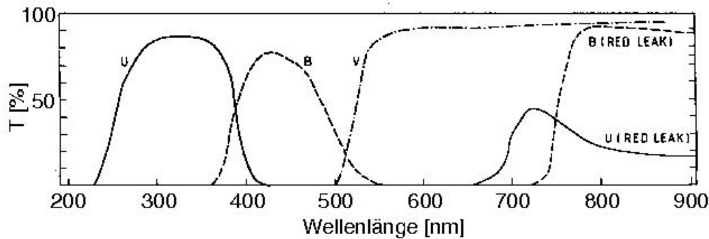
Abb. 7.17 Spektrale Durchlässigkeiten für UBV-Filter. Der original V-Filter ist ein Langpassfilter. Man beachte bei dem U- und B-Filter die Durchlässigkeit (red leak) im Infraroten, welche beim Einsatz einer CCD beachtet werden muß. Mit freundlicher Genehmigung von Kluwer Academic Publishers
