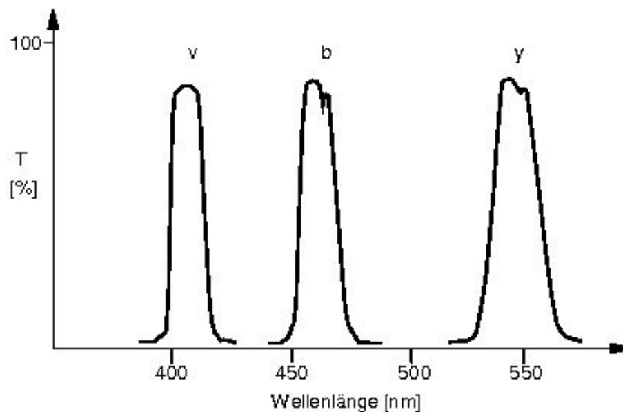
Abb. 7.21 Transmissionen der Strömgren vby-Filter. T: Transmission
