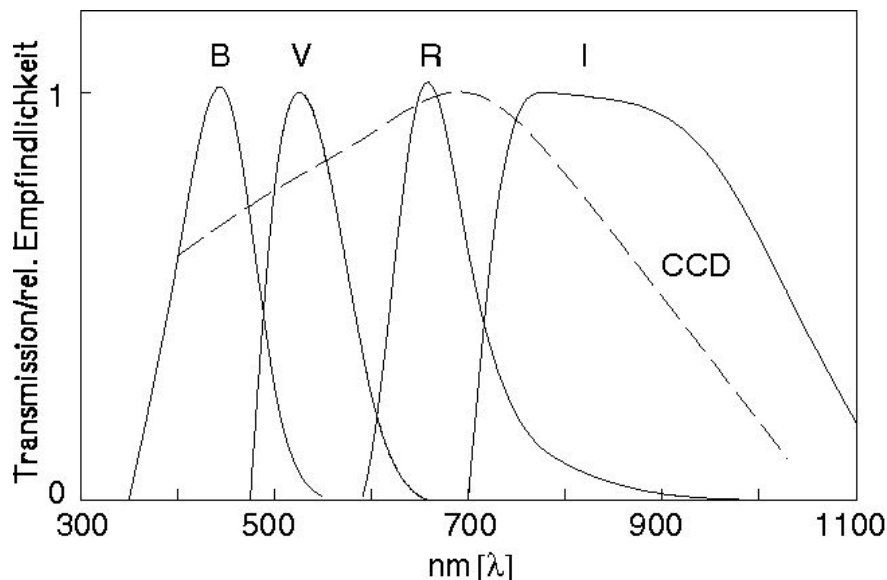
Abb. 7.18 Schematische Darstellung normierter Transmissionskurven der BVRI-Filter im Kron-Cousins-System. Das I-Band wird rechtsseitig durch die spektrale Empfindlichkeit der CCD bestimmt
