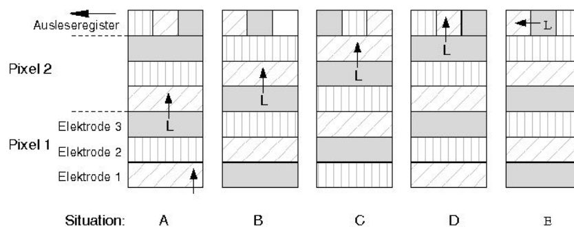
Abb. 7.8 Dreiphasentransfer entlang einer Zeile von einem Pixel zum nächsten Pixel (Situation A-D) und ein Transferschritt entlang dem Register (Situation E)
