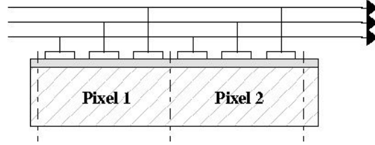
Abb. 7.7 Kopplung gleichartiger Elektroden bei einem Dreiphasentransfer
