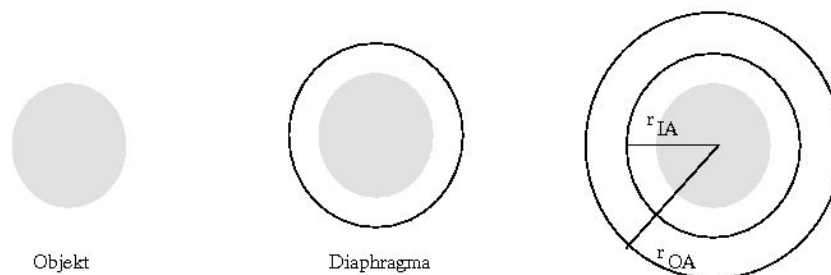
Abb. 7.25 Diaphragma-Methode der Aperture-Photometrie zur Bestimmung des Signals eines Objektes. r_{IA} und r_{OA} sind die Meßkreisradien zur Himmelshintergrundkorrektur
