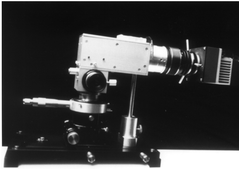
Abb. 9.6 Ansicht des im Text beschriebenen Spaltspektrographen, "huckepack" montiert auf einem 300 mm f/4.8 Newton der Sternwarte an der Universität-Gesamthochschule Siegen. Man erkennt unten den Okularschlitten, auf dem sich z.Zt. noch ein Feintriebokularauszug befindet. Aufgesetzt ist der Spektrograph. Nach links ragt die Mikrometerschraube für den verstell- und drehbaren Spalt heraus. Rechts erkennt man (blau) die angesetzte CCD-Kamera vom Typ LcCCD11n (Fa. OES).
