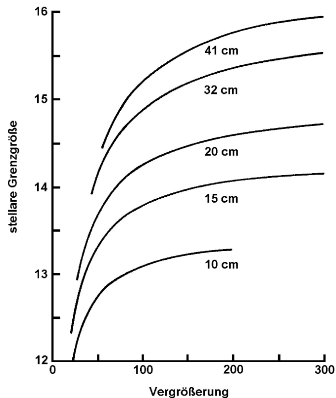
Abb. 3.3 Visuelle stellare Grenzgrößen bei unterschiedlichen Teleskopöffnungen und Vergrößerungen. Aus Schaefer (1989)
