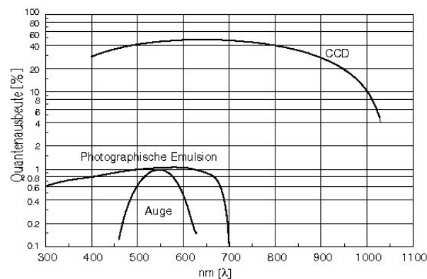
Abb. 7.10 Quantenausbeute verschiedener Detektoren
