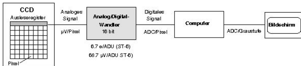
Abb. 7.9 Analog/Digital-Wandlung bei der ST-6
