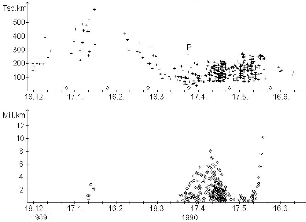
Abb. 5.10 Zeitliche Entwicklung des absoluten Komadurchmessers und der absoluten Schweiflänge beim Kometen Austin (1990 V)
