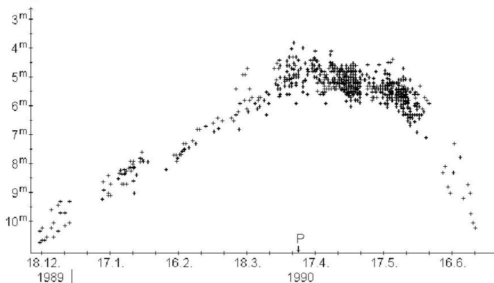
Abb. 5.2 Zeitliche Entwicklung der Gesamthelligkeit des Kometen Austin (1990 V). Das Diagramm enthält alle erfaßten Schätzungen.
