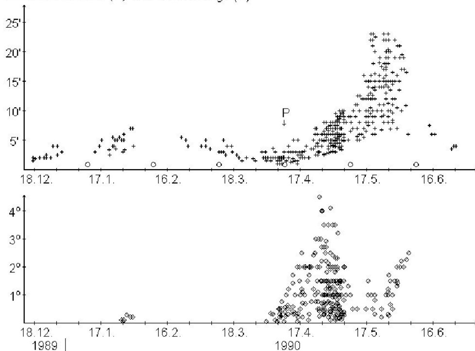
Abb. 5.9 Zeitliche Entwicklung des scheinbaren Komadurchmessers und der scheinbaren Schweiflänge beim Kometen Austin (1990 V)
