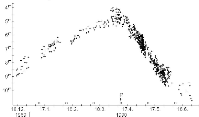
Abb. 5.7 Die heliocentrische Helligkeit des Kometen Austin (1990 V), aufgetragen über dt
