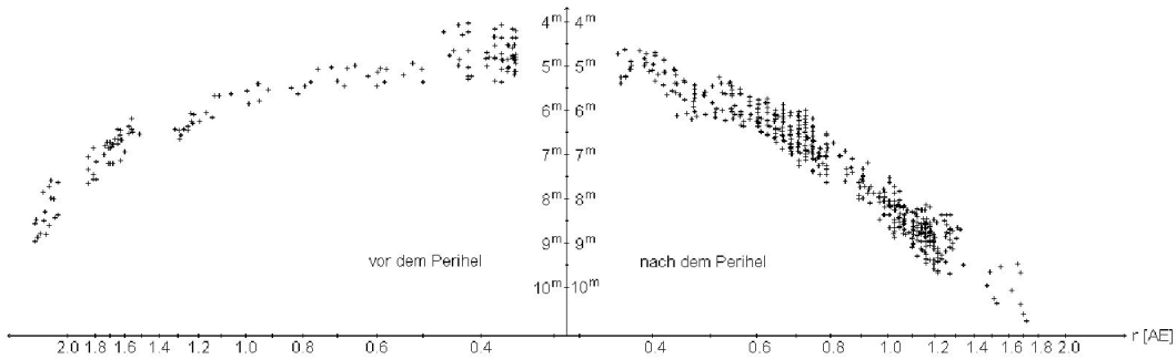
Abb. 5.6 Die heliocentrische Helligkeit des Kometen Austin (1990 V), aufgetragen über \log r
