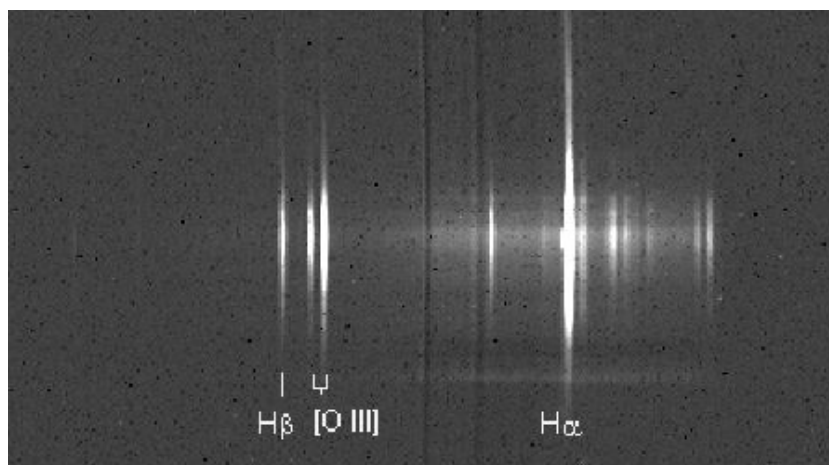
Abb. 9.7 CCD-Spektrum des Orionnebels (M42), aufgenommen am 14.10.1996, 3:23–3:33 UT mit 300 mm f/4.8 Newton und LcCCD11n (KAF-0400 im 2 \times 2 -Binning-Mode). Die Spaltweite am Himmel betrug 22'' . Aufnahme: M.Jung & M.Kretlow (Siegen).
