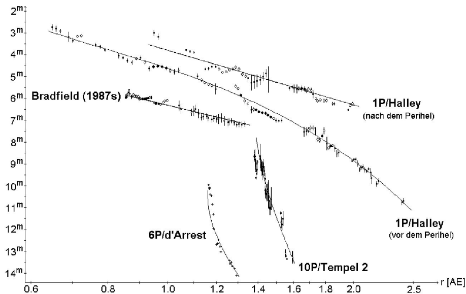
Abb. 5.4 Die heliozentrische Helligkeit von vier ausgewählten Kometen, aufgetragen über \log r (bzgl. Interpretation siehe Abb. 5.5)
