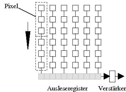
Abb. 7.4 Zeilenweiser Aufbau des Sensor-Arrays
