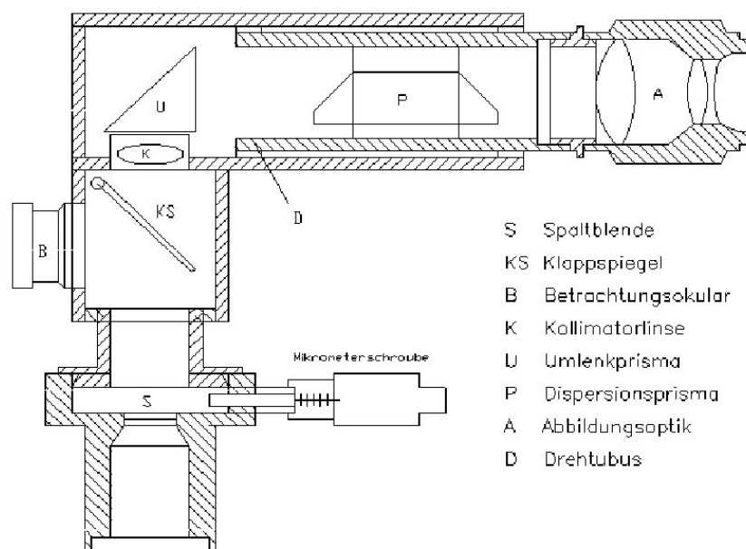
Abb. 9.4 Aufbau eines für den Selbstbau geeigneten Spaltspektrographen mit Geradsichtprisma als Dispersionselement. Die abgewinkelte Anordnung ergibt sich aus Stabilitätsgründen am Okularauszug, sie ist aber nicht zwingend. Zu den Details der einzelnen Baugruppen siehe Text und Bildunterschrift des aufgenommenen Kometenspektrums. Skizze und Konstruktion: K.-H.Uhlmann (Lampertheim), M.Jung & M.Kretlow (Siegen).
