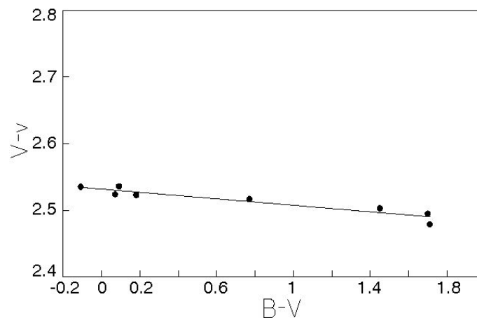
Abb. 7.24 Bestimmung der Transformationskoeffizienten für das V-Band
